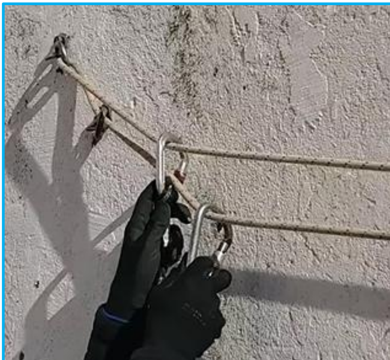
Ilustración 29. Colocación de las bagas de anclaje para progresión por el pasamanos recuperable.
