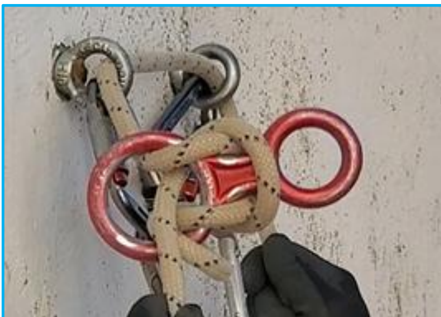
Ilustración 24. Ocho en retención con llave peinada montado en lado contrario a la bajada
