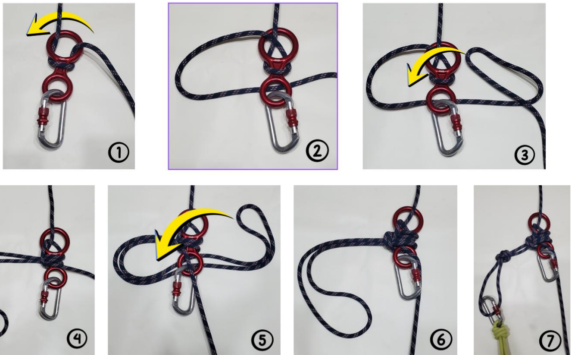
Ilustración 22a. Llave de bloqueo del descendedor tipo ocho. Montaje en clásico
