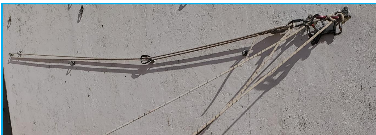
Ilustración 30. Instalación completa de pasamanos recuperable con punto intermedio y cabecera recuperable.
